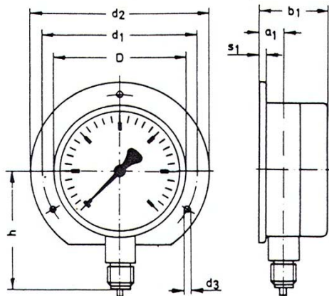
Tilslutning nedad med bagflange
