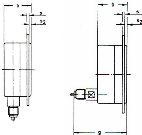
Tilslutning bagud med frontflange
